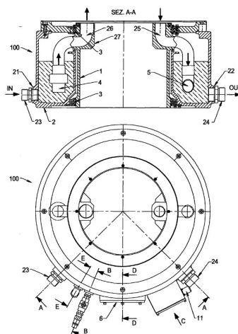
Figura 1. Struttura meccanica del giunto idraulico
