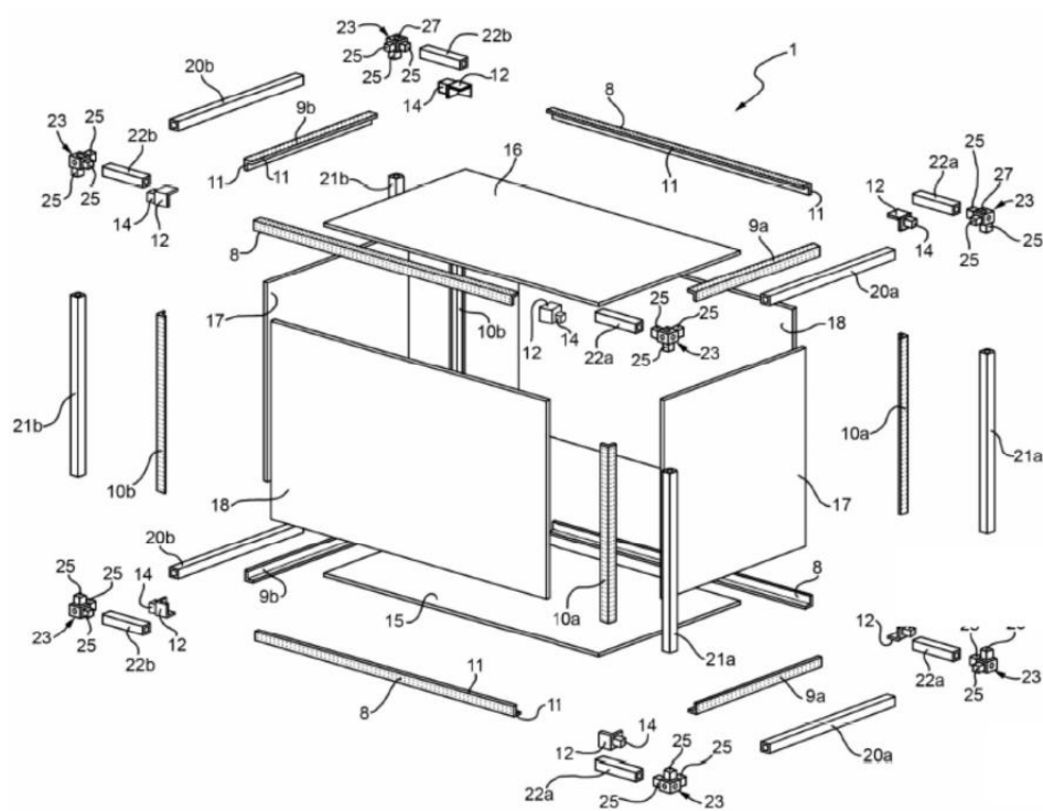
Figura 2. Elementi base principali costituenti lo shelter
