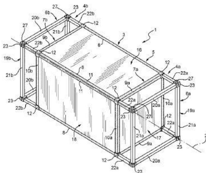
Figura 1. Realizzazione dello Shelter sulla base della soluzione esposta dal brevetto
