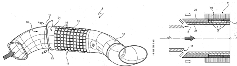
Figura 1 - Installazione dei moduli sugli scarichi (disegno a sinistra) e mantenimento del gradiente tramite flussi / dissipatori (disegno a destra)
