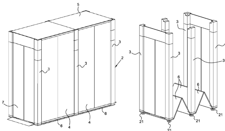
Figura 1 – Visione d'insieme del modulo di identificazione controllo accessi e suo ripiegamento
