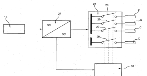
Figura 2 - Implementazione tramite DC/DC converter, barra di alimentazione dedicata e sezionatori
