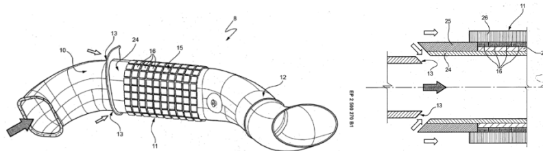
Figura 1 - Installazione dei moduli sugli scarichi (disegno a sinistra) e mantenimento del gradiente tramite flussi / dissipatori (disegno a destra)
